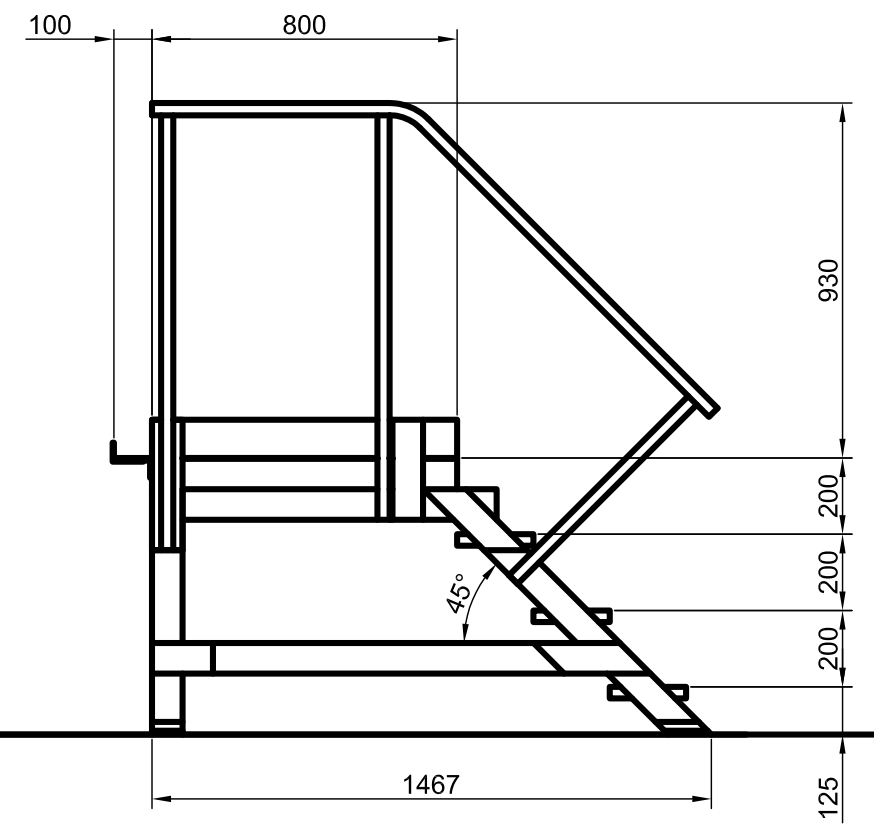
CORTE A-A
