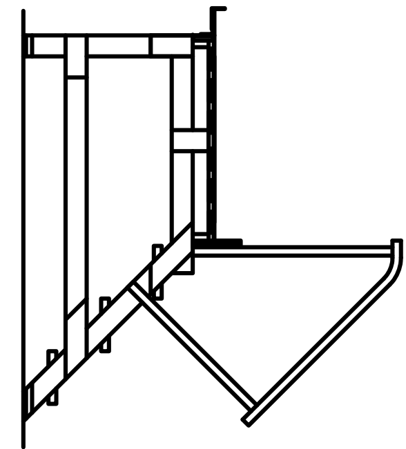
CORTE A-A
